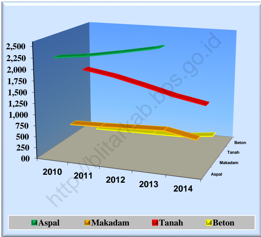
Gambar : 8.1.1 Panjang Jalan Kabupaten Menurut Jenisnya, 2010-2014 Figures Length of Regency Road by Kind, 2010-2014 (Km)
